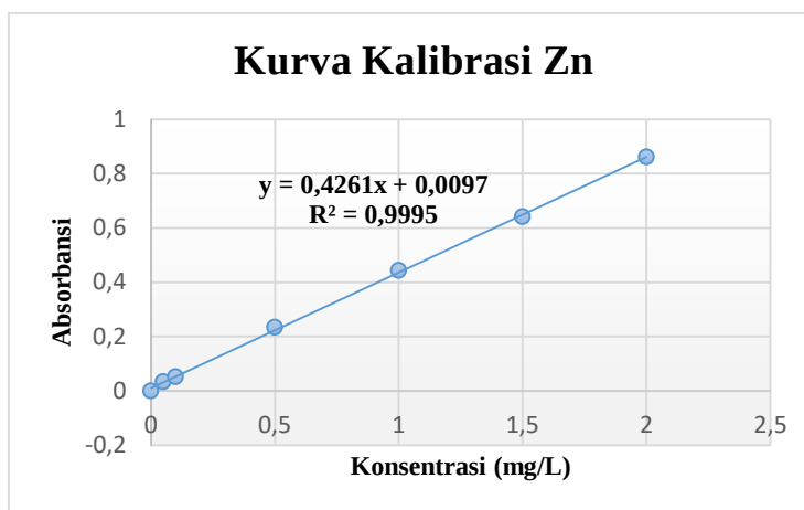
Gambar 2. Kurva Kalibrasi Larutan Standar Logam Zn
